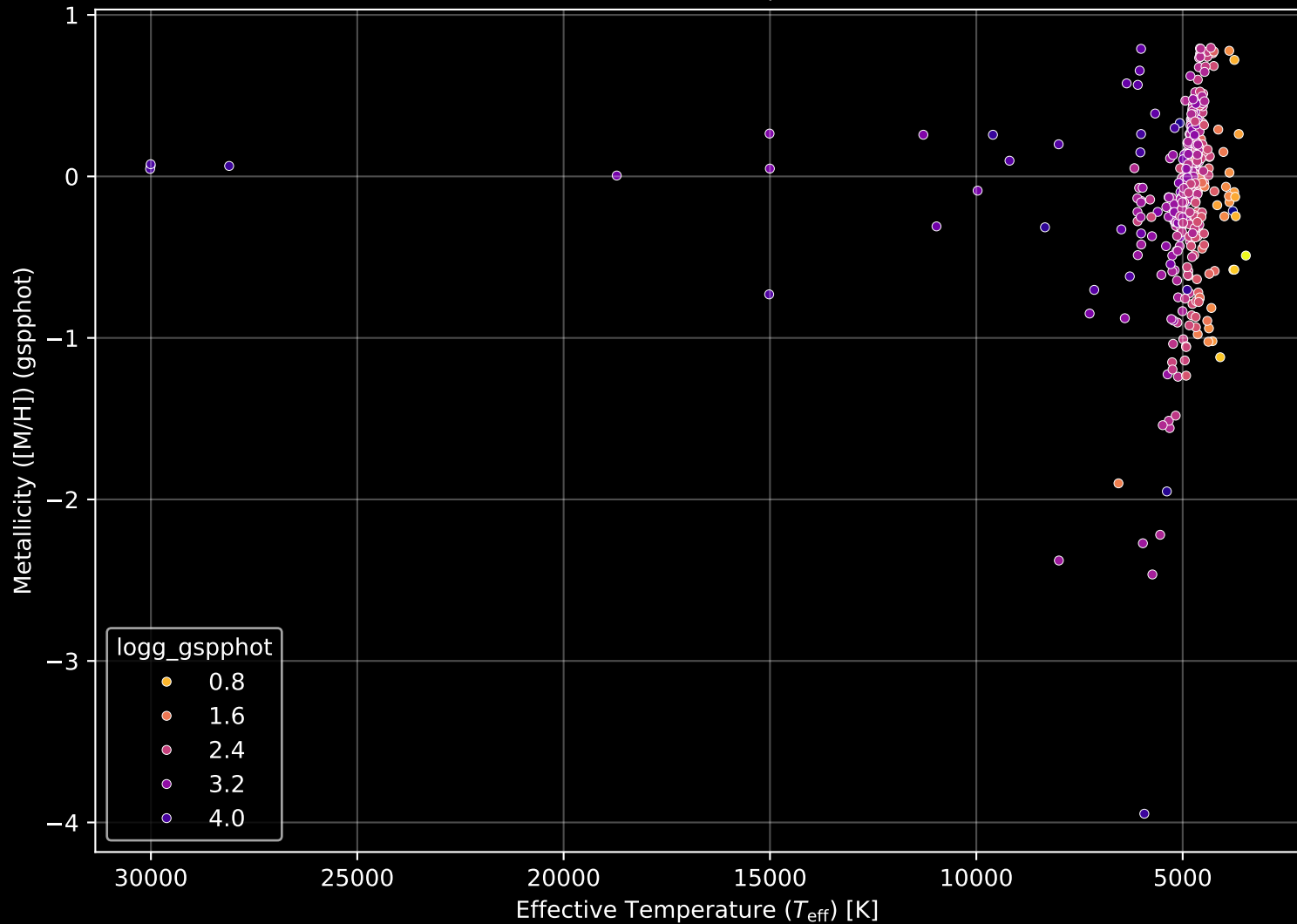
APOGEE DR17 Field: [003-03-C] Stellar Population Parameters (n= 392)
